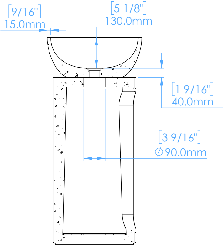
Section A-A
